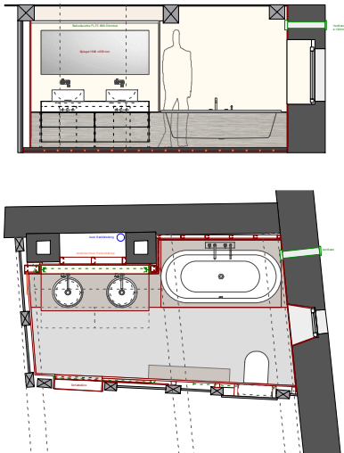
Innenansicht und Grundriss Badezimmer 1/100
