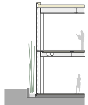
Ausschnitt Querschnitt 1/200
