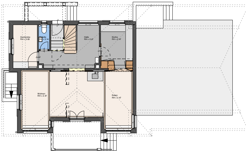
Erdgeschoss 1/200
